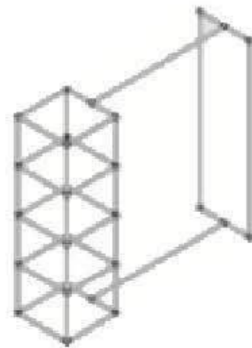
L-16 Yükseklik: 130 cm Genişlik: 140x39 cm Cam Ölçü: 34.7x34.7 cm / 5 adet
