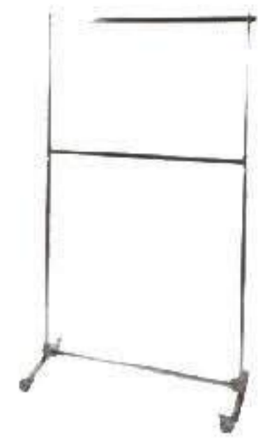
TD-10 - Elips Süper Çift Katlı Profil : □ 20x40 mm Genişlik : 120 cm Uzunluk : 220 cm Renk : Krom, Gümüş
