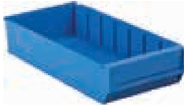
SV-419 Ebat / Size En / W Boy / L Yük / H Dış / Ext 188 400 80 mm
