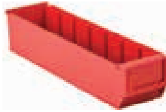
SV-409 Ebat / Size En / W Boy / L Yük / H Dış / Ext 90 400 80 mm
