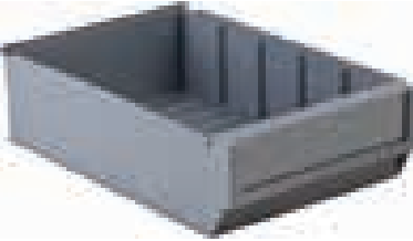
SV-319 Ebat / Size En / W Boy / L Yük / H Dış / Ext 188 300 80 mm
